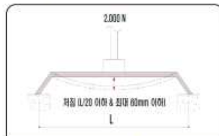
단면도 (성능기준: 처짐)
