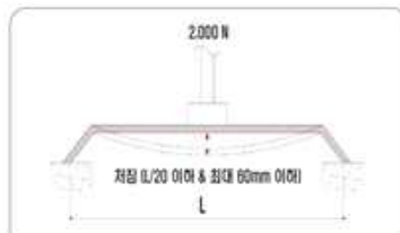
단면도 (성능기준: 처짐)
